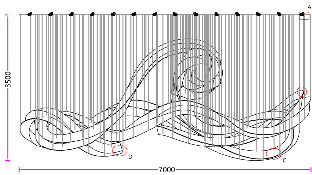
主视图/Front View
