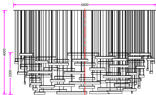
主视图/Front View
