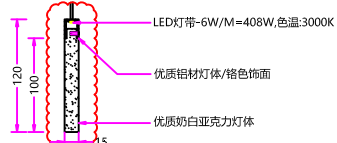
B 部细节图/Part B Details
